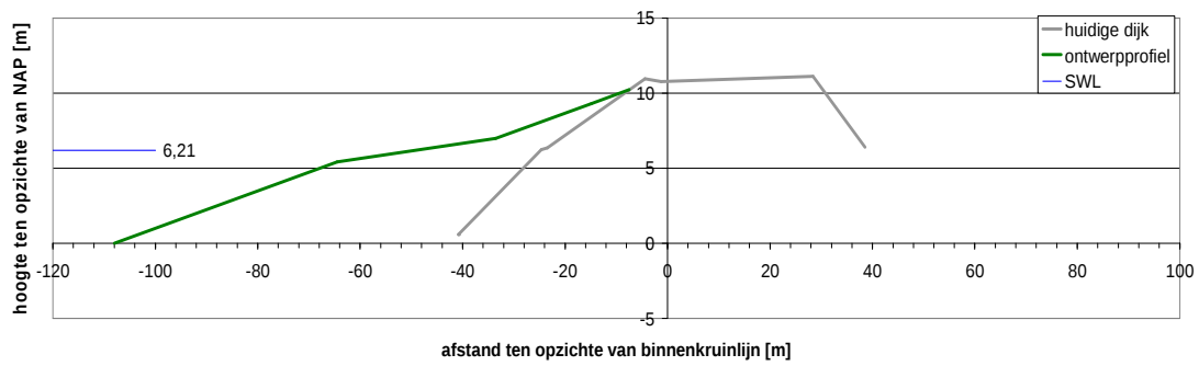
ontwerpprofiel dijkversterking Breskens Veerhaven Oost op basis van km raai 68,000
