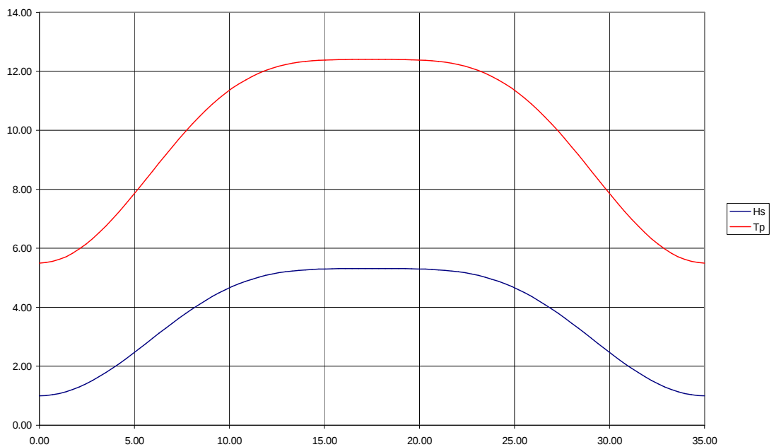
verloop van de golfrandvoorwaarden gedurende de storm
