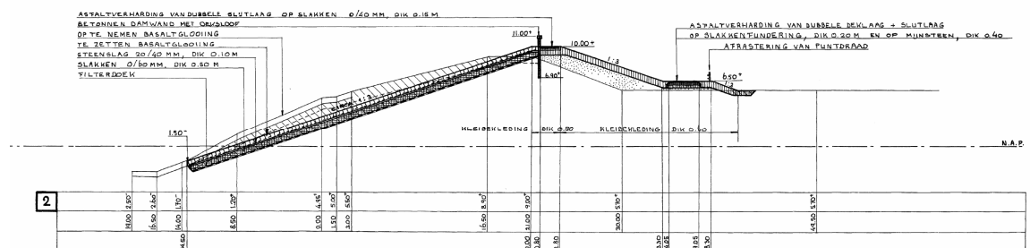
Doorsnede IV (oranje); bron: profiel 2 van Kievitte Oost 1987
